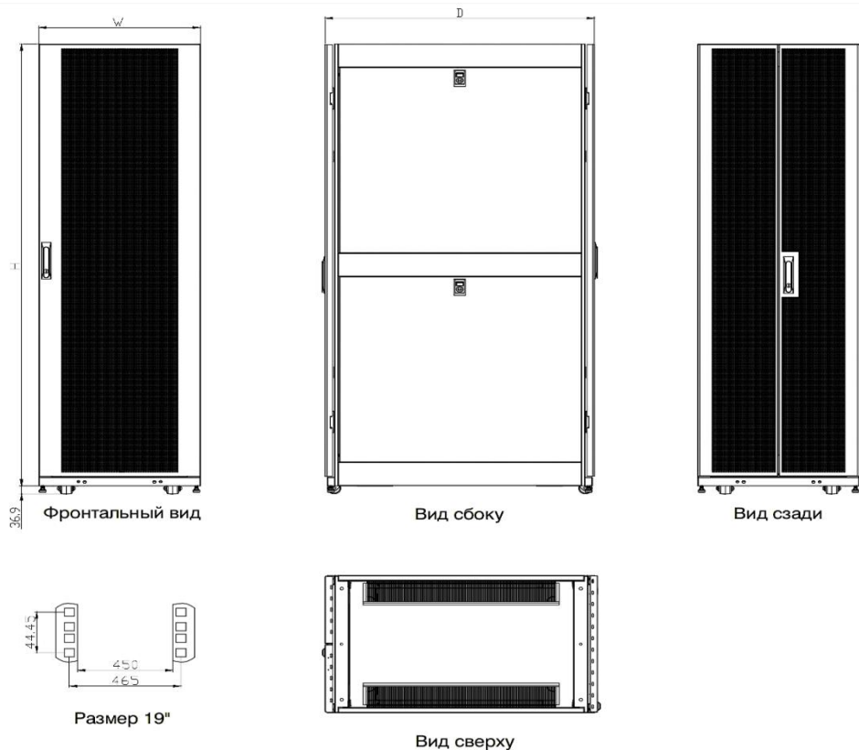
Рисунок 3 - Габаритные размеры шкафа
