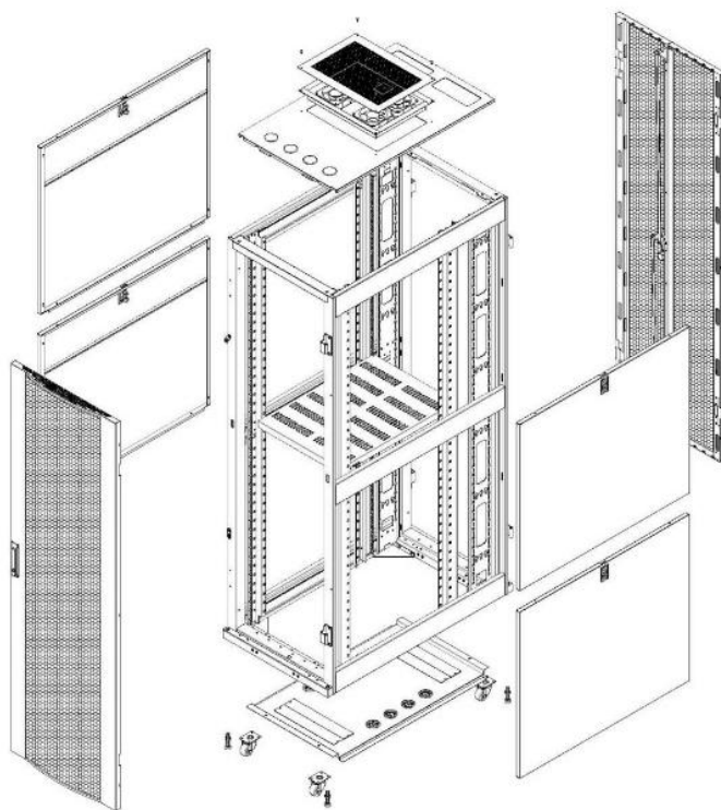
Рисунок 1 – Комплектация шкафа
