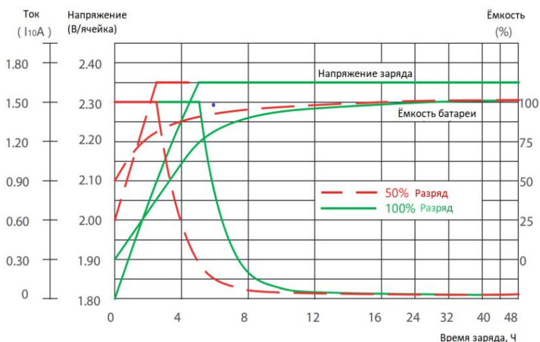
Характеристики заряда при постоянном напряжении (при 25°C)
