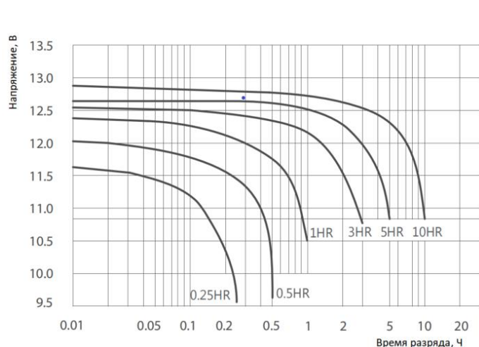
Зависимость напряжения от времени разряда
