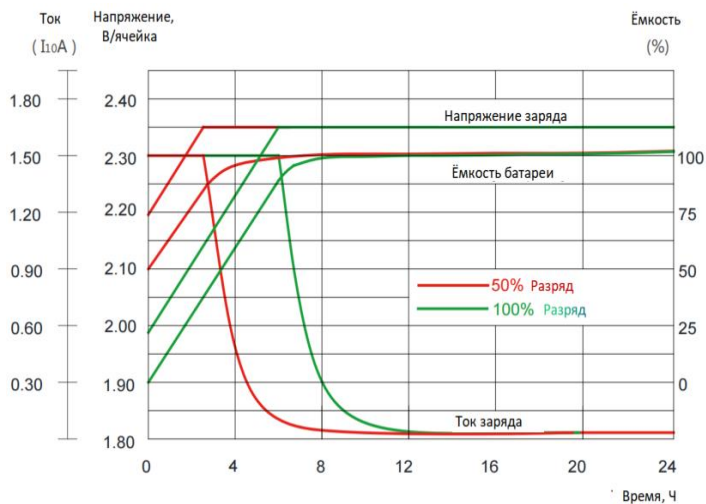
Характеристики заряда при постоянном напряжении (при 25°C)
