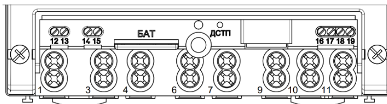
а) обозначение контактов счетчика с интерфейсом EIA-485
