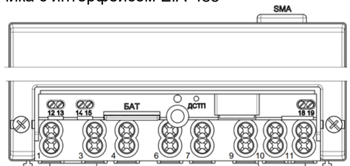
г) обозначение контактов счетчика с радиомодулями, с внешней антенной
