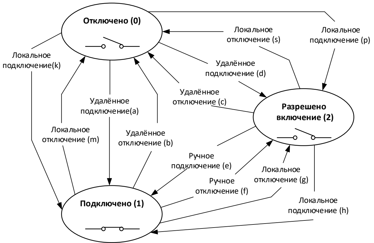
Рисунок 140 – Возможные переходы реле
