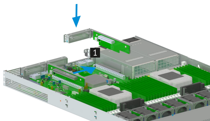
Рис. 46. Установка PCIe-райзера с основанием в корпус сервера
