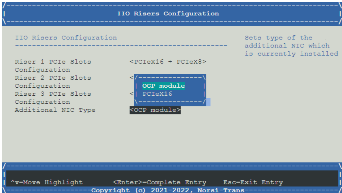
Рис. 64. Меню IIO Risers Configuration
