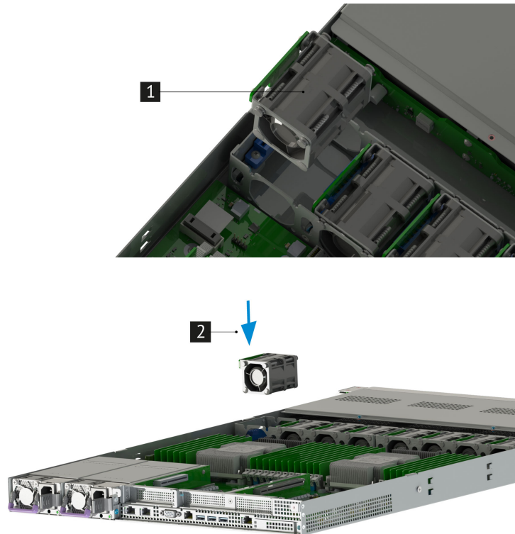
Рис. 29. Подключение вентилятора
