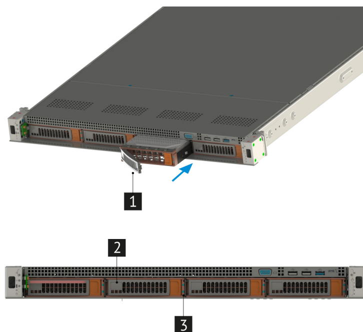
Рис. 42. Извлечение дисков
