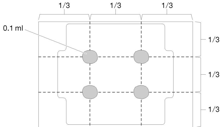
Рис. 36. Нанесение термопасты
