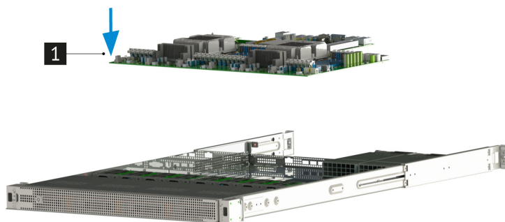
Рис. 39. Установка материнской платы
