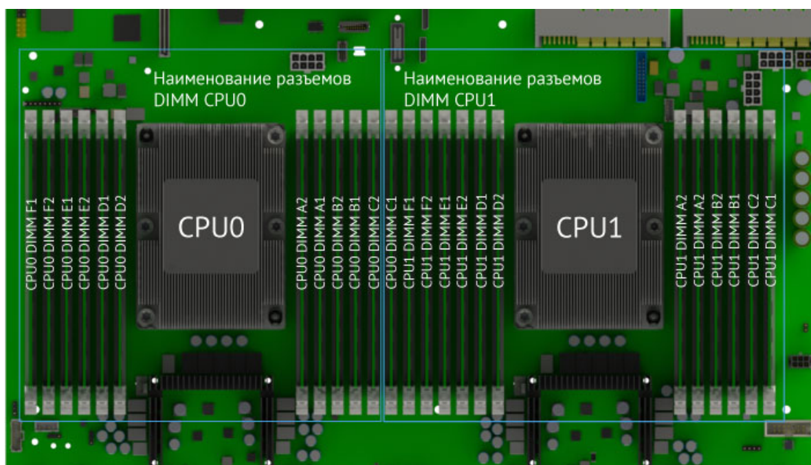
Рис. 30. Расположение разъемов
