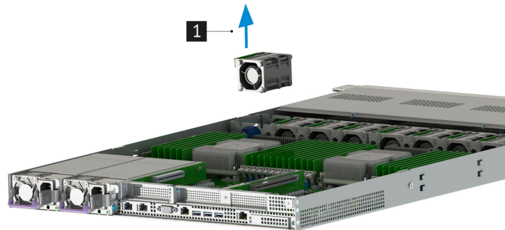
Рис. 28. Извлечение вентилятора
