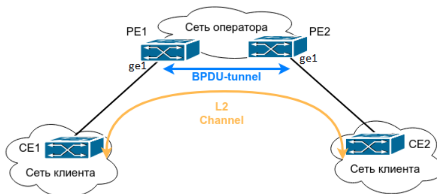
Рис. 9: BPDU-Tunnel
