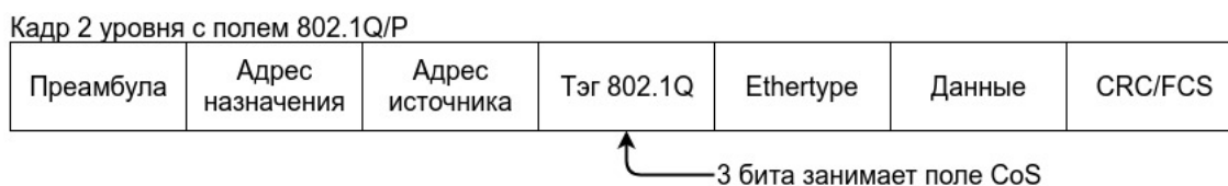
Рис. 18: Поле CoS
