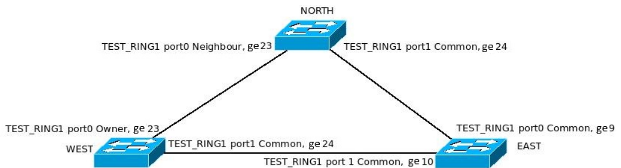
Рис. 16: Топология ERPS
