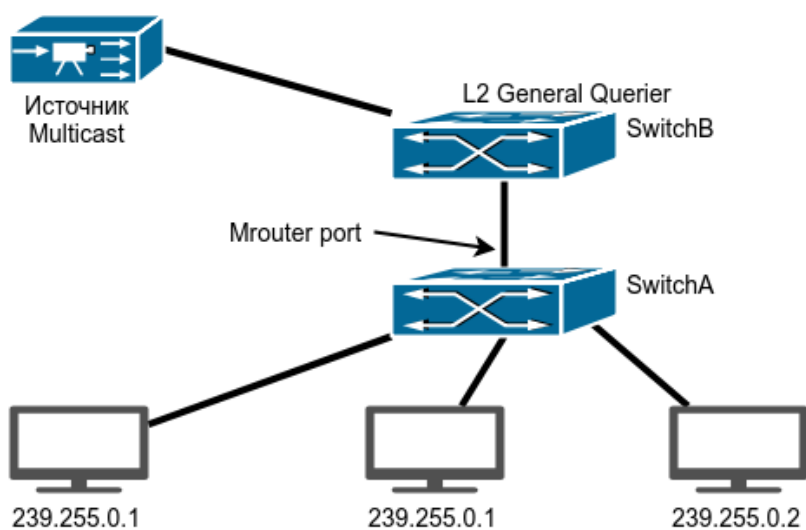
Рис. 31: IGMP Querier
