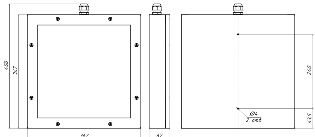
Рис. №2 Габаритный чертёж.
